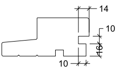
Cill groove type 26
