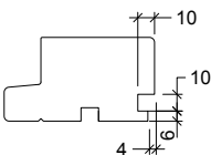
Cill groove type 6
