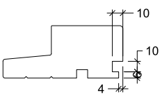
Cill groove type 6
