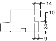
Cill groove type 5
